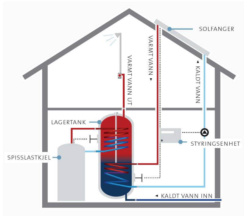
Figur 5. Prinsippkisse av et solvarmeanlegg til oppvarming av forbruksvann (figuren viser ikke reelle forholdsmessige størrelser på tank, kjel, osv). Illustrasjon: Tibe-T.
