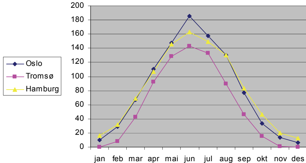
Figur 1. Månedlig total solinnstråling på horisontalen (W/m 2 ) for Oslo, Tromsø og Hamburg. Data for solinnstråling er basert på målte gjennomsnittsverdier over 20 år.
